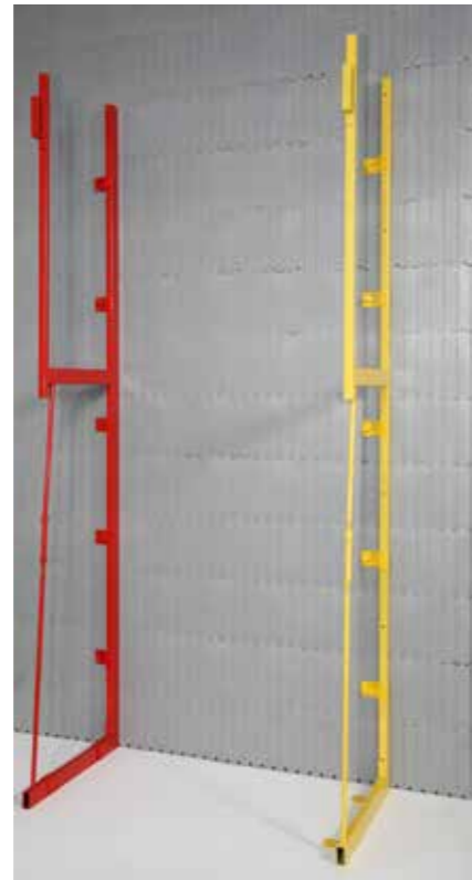
Die Stahlstützen erleichtern den Aufbau der Wand, die Kontrolle der Ebenen mit dem Erhalten des Vertikalen. Die Stützen mit roter Farbe sind für die Montage des Aufsatzes mit einer Höhe von 110 cm geeignet.
