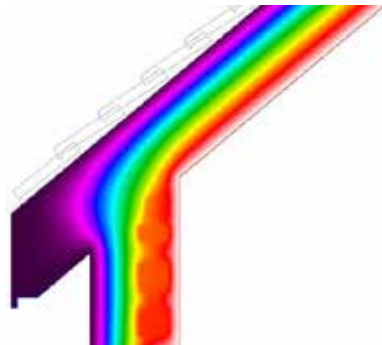
Die Abbildung zeigt einen sehr guten thermischen Schutz, welchen die Anwendung des Elementes MP beim Bau eines Kniestocks gewährleistet. Die Kontinuität der Isolierschicht schützt das Gebäude vor Wärmeverlusten und Feuchtigkeit.
