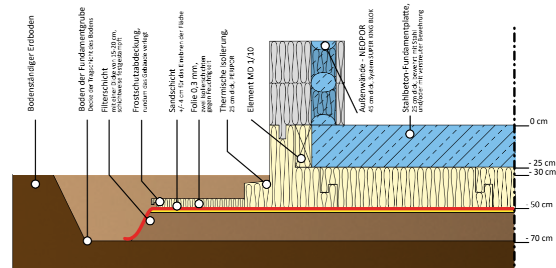
Abb. 1 Schema der Fertigung des Plattenfundaments in der Version mit den Außenwänden einer Breite von 45 cm (Super King Blok)
