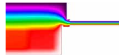
Die Abbildung zeigt, wie die sog. warme Montage des Fensters vor dem Eindringen der Kälte schützt.
