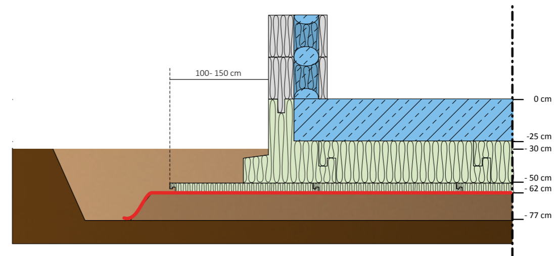
Abb. 2 Schema der Fertigung des Plattenfundaments mit der Anwendung einer zusätzlichen thermischen Isolierung.
