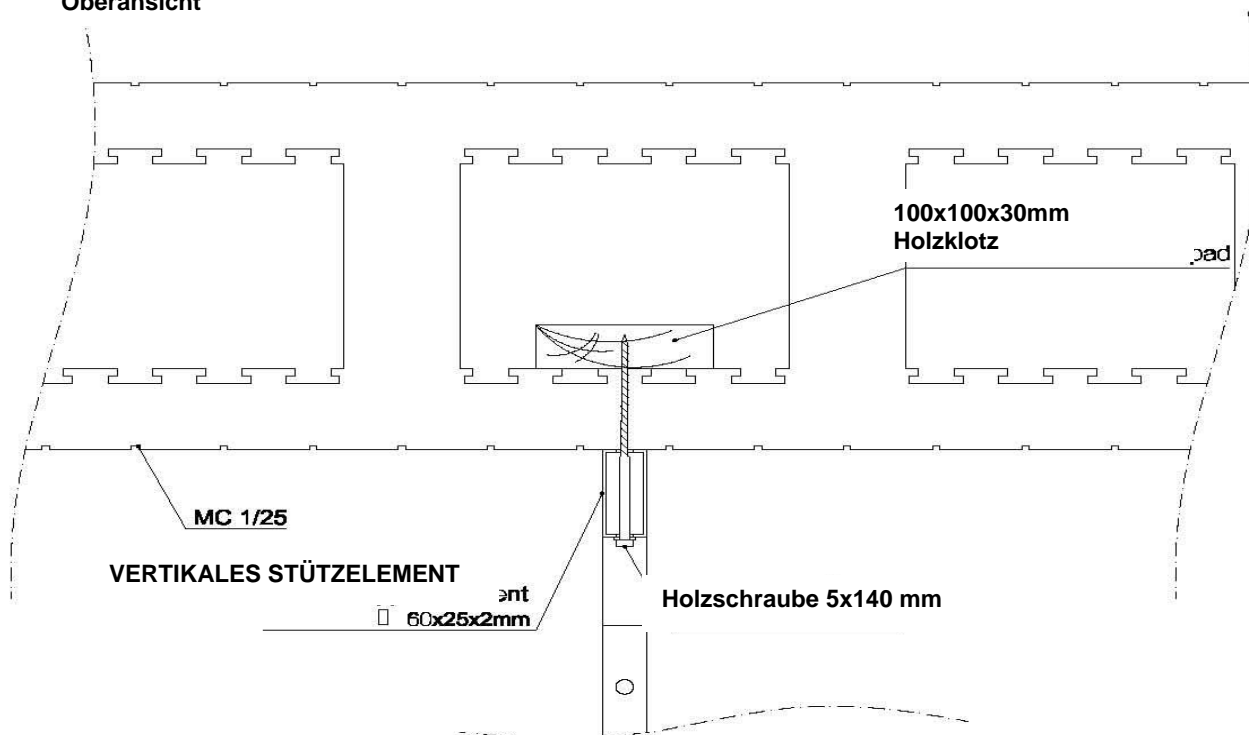
Oberansicht
