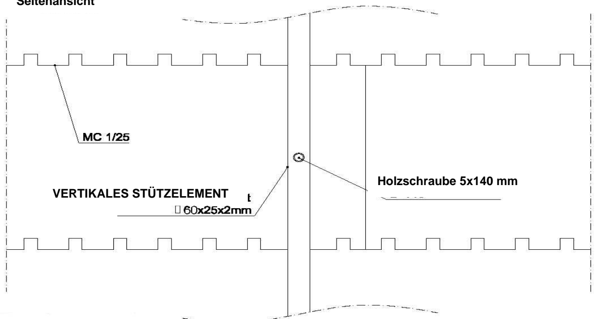
Seitenansicht
