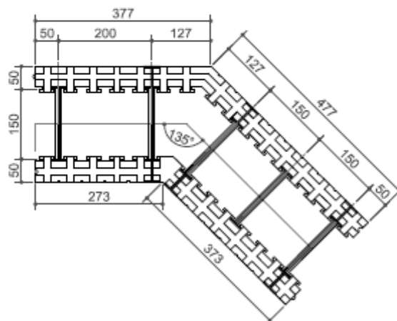
DRAUFSICHT
