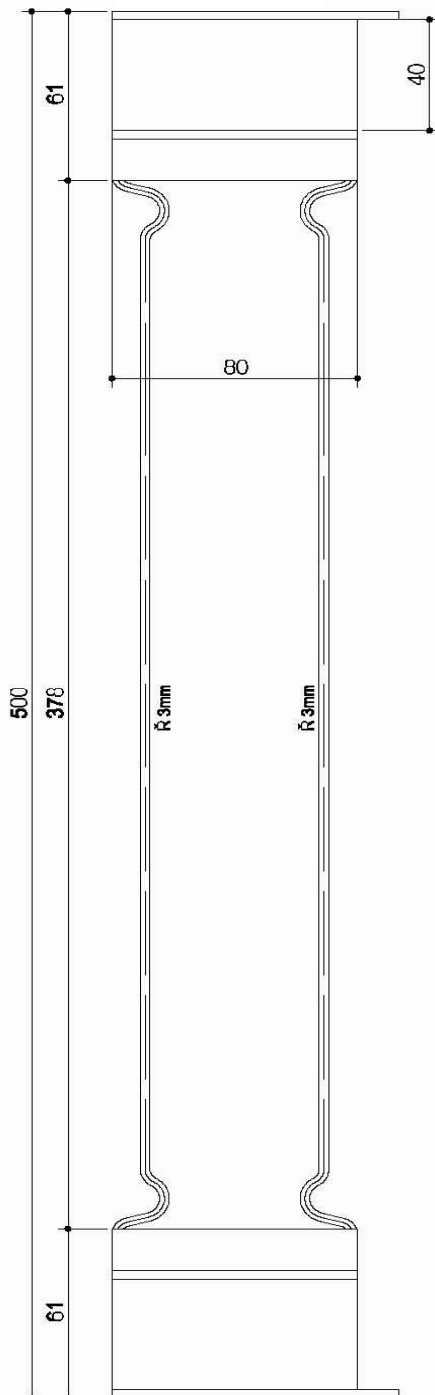
Seitenansicht
